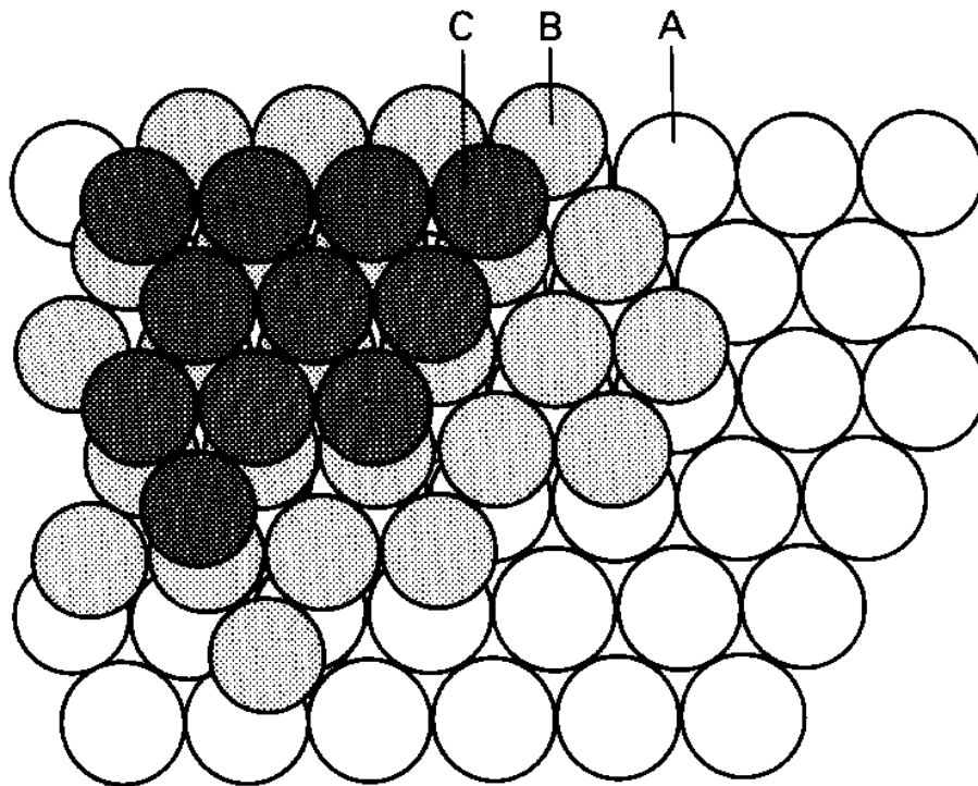
Cubic
